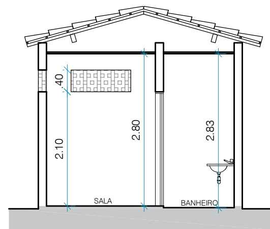
CORTE AA
